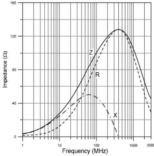
CB 1608-101
