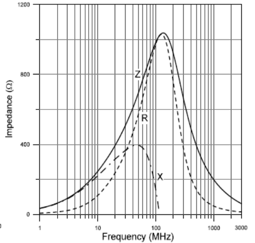
CB 1608-102
