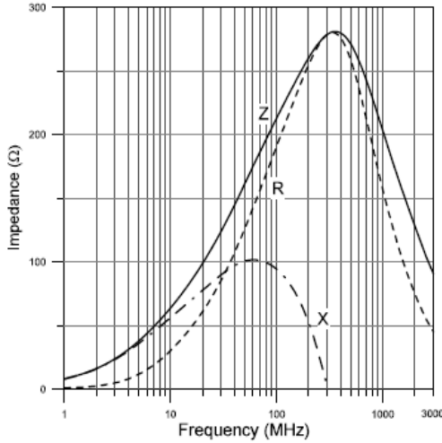
CB 1608-221
