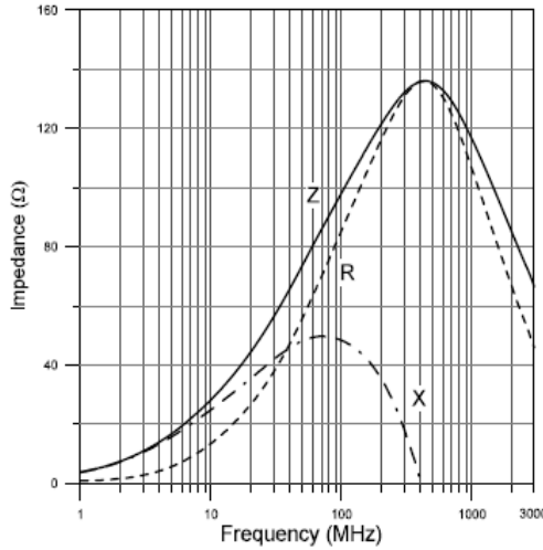
CB 1608-121
