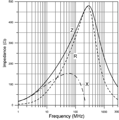
CB 1608-301
