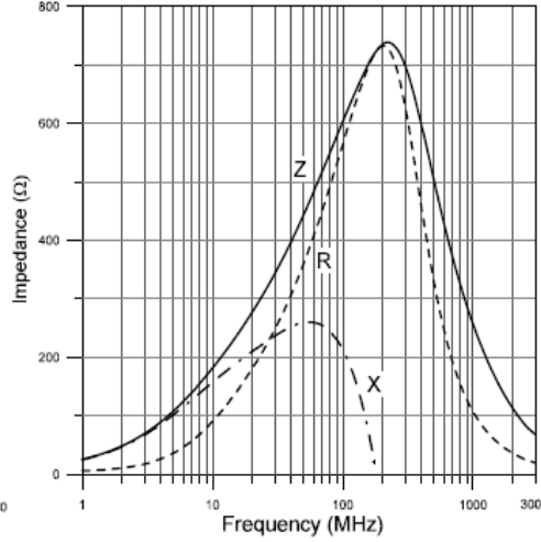
CB 1608-751
