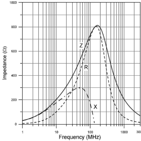
CB 1608-601
